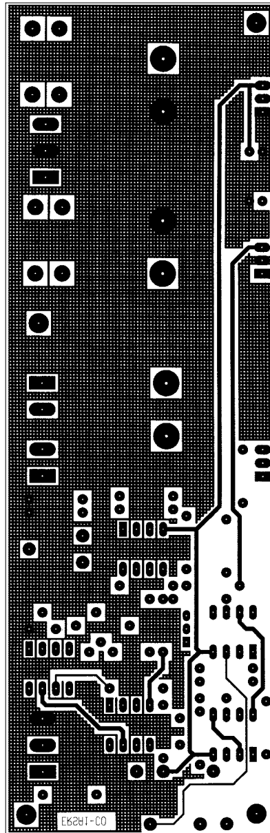
Bild 7: Oberseite der beidseitig beschich-ten Platine
