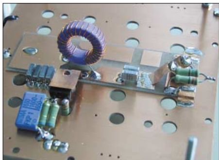
Bild 5: Messaufbau eines einzelnen Verstärkers gemäß Bild 2 ohne Parallelkompensation und Schutzbeschaltung; Ausgangsseite, Kühlkörper demontiert.
