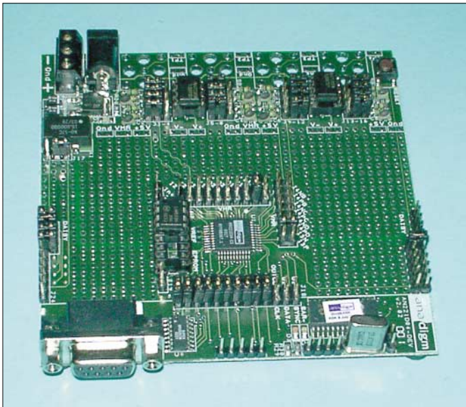
Bild 1: Das Starterkit von Anadigm erleichtert preiswert den Einstieg in die neue FPAA-Technik.
