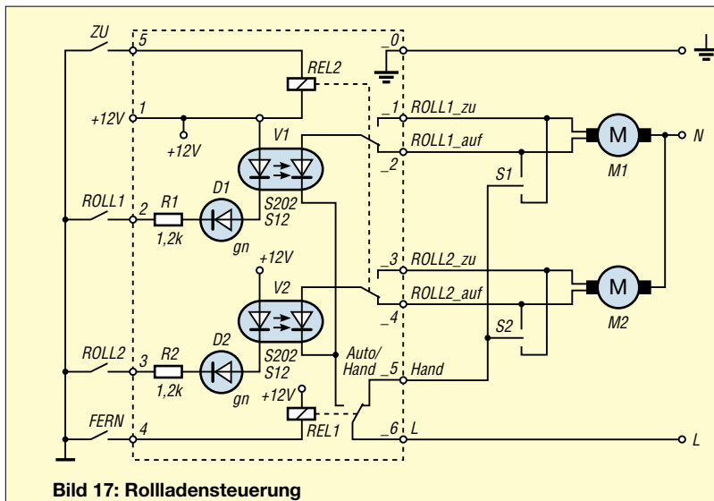
Bild 17: Rollladensteuerung
