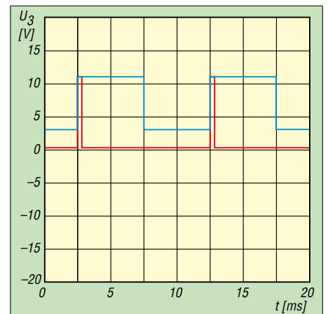
Bild 4: Je nach eingestellter Temperatur gibt IC3 bei niedrigen Werten kurze (rot) und bei hohen Werten lange Heizimpulse (blau) ab.
