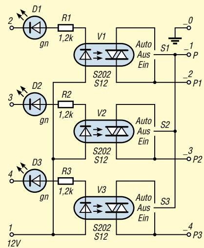
Bild 18: Beleuchtungs- und Lüftersteuerung
