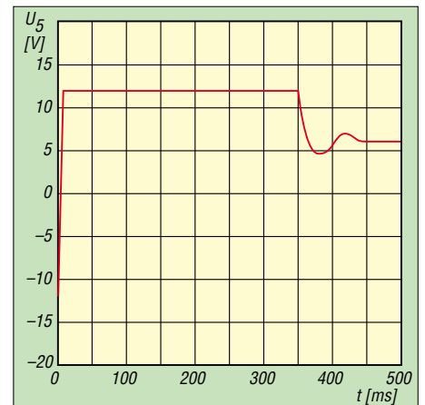
Bild 5: Das Einschwingverhalten der Regelung, hier nach 350 ms, lässt sich durch Variieren von R23 beeinflussen.
