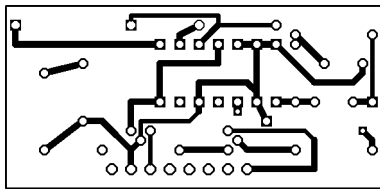
Bild 24: Layout des Windstärkesensors
