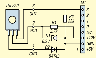
Bild 22: Im Lichtsensor erzeugt die Zener-Diode einen Offset, um so Codewerte unter 4 zu umgehen.
