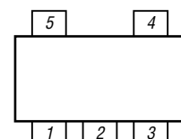
Bild 2: Pinbelegung (SOT23)
