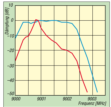
Bild 3: Frequenzgang des CW-Filters zusammen mit einem SSB-Filter älterer Bauart
