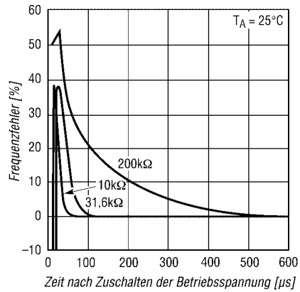
Bild 4: Ausgangsfrequenzfehler nach Zuschalten der Betriebsspannung bei unterschiedlichen Setzwiderständen
