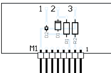
Bild 27: Bestückung des Lichtsensors
