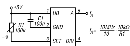
Bild 7: Temperatur-Frequenz-Umsetzer
