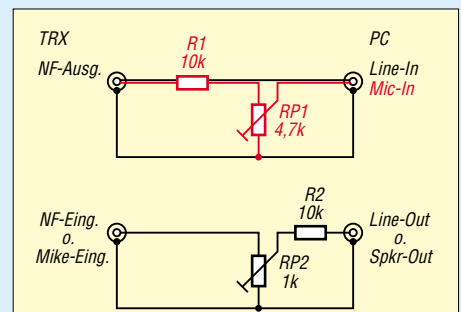
Bild 2: Verbindung zwischen Transceiver und Soundkarte
