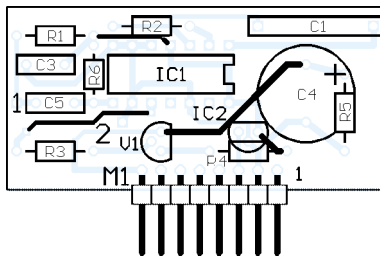
Bild 25: Bestückung des Windstärkesensors
