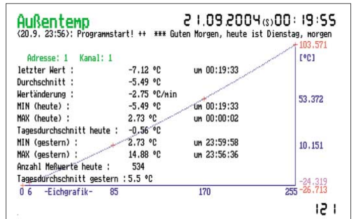
Bild 30: Im Datenlogger sind die Spannungsverläufe des Helligkeits-sensors und der drei Temperatü-fer zu erkennen.
