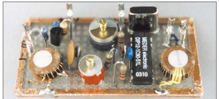
Bild 5: Aufbau des erweiterten Filters Fotos: DL7HG
