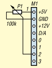
Bild 23: Mechanischer Winkelsensor
