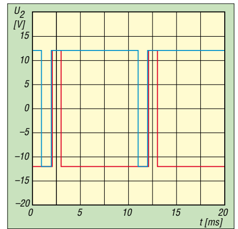
Bild 3: Ausgangsspannung an IC2 bei voller Heizleistung (blau) und nach dem Erreichen der eingestellten Temperatur (rot)
