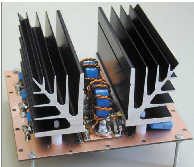
Bild 1: Ausgangsseite eines fertig aufgebauten 250-W-Verstärkers auf einer 12 \times 13 \text{ cm}^2 großen Platine; unter den Kühlkörpern befinden sich je drei Transistoren.
