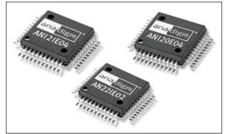
Bild 2: Alle FPAA-Schaltkreise werden mit QFP-Gehäuse hergestellt.
