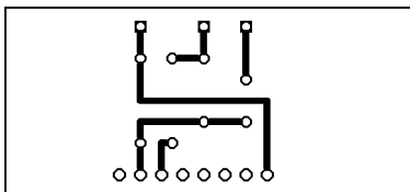
Bild 26: Layout des Lichtsensors
