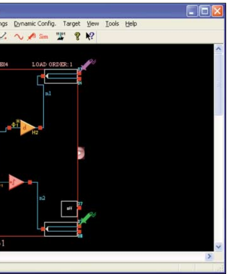
Bild 7: Das vom virtuellen Signalgenerator kommende Rechtecksignal wird differenziert, integriert und mit dem Oszilloskop betrachtet.
