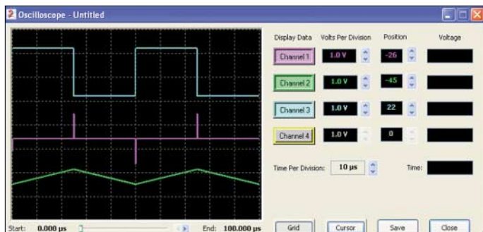
Bild 5: Mit dem virtuellen Oszilloskop lässt sich die Funktion der Schaltung überprüfen.
