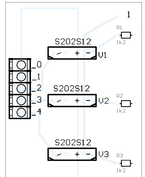
Bild 29: Bestückung der Schaltstufe für Beleuchtung und Lüfter
